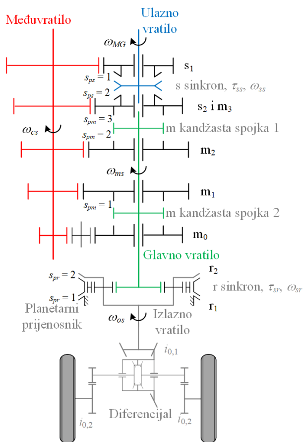
Slika 2-5. Shematski prikaz razmatrane automatizirane manualne transmisije (AMT) s 12 stupnjeva prijenosa te prigranskog sklopa [91].
