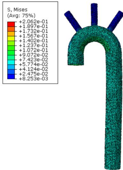
Slika 48. Raspodjela naprezanja u modelu za početni trenutak (pogled za točku 3)
