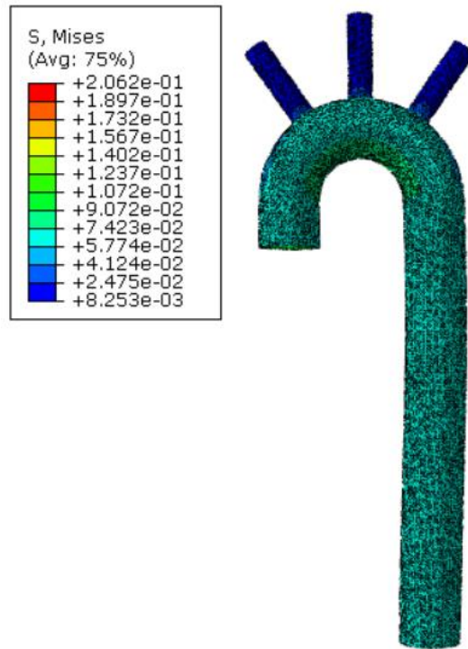
Slika 48. Raspodjela naprezanja u modelu za početni trenutak (pogled za točku 3)
