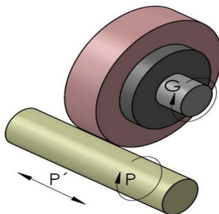
Slika 2-3 Okruglo vanjsko uzdužno brušenje [7]
