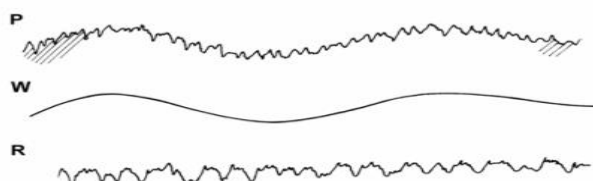
Slika 6-2 Razlučivanje P, W i R karakteristika profila [29]
