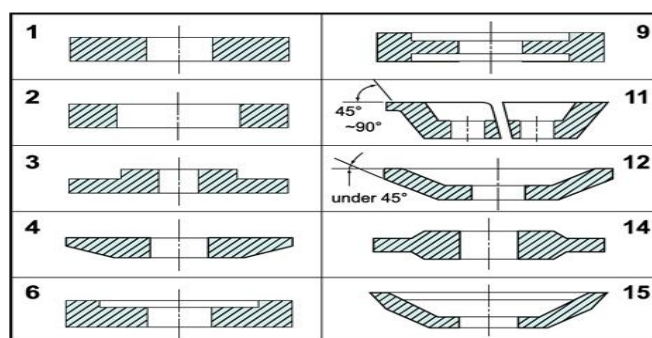
Slika 4-2 Oblici brusnih ploča [32]
