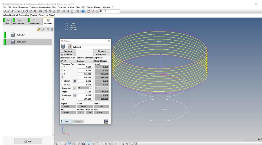
Slika 7-15 Trajektorija ticala
