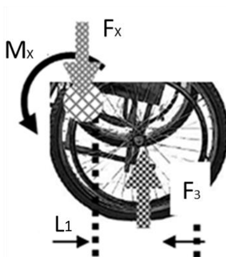
Slika 26. Prikaz opterećenja „X“ dijela okvira invalidskih kolica [21]
