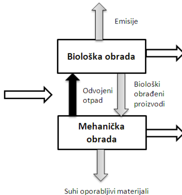
Slika 2.13. Opća shema MBO procesa s obzirom na redoslijed obrade [7]
