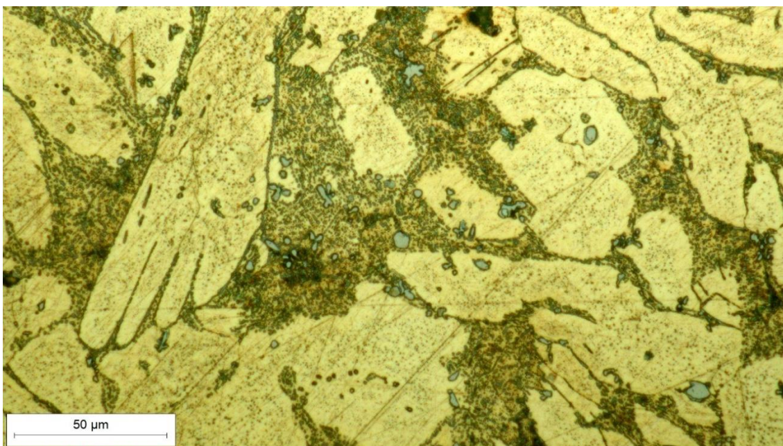
Slika 24. Osnovni materijal u nagriženom stanju, snimljeno pri povećanju 500×
