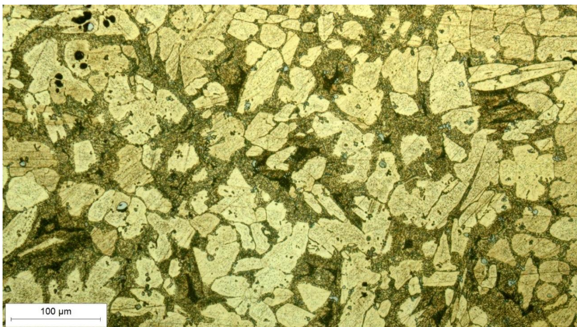
Slika 23. Osnovni materijal u nagriženom stanju, snimljeno pri povećanju 200×
