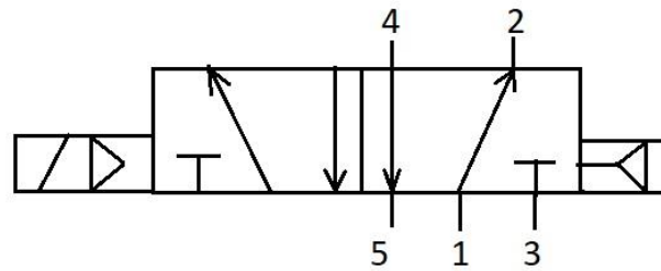
Slika 15. Simbol pneumatskog razvodnog ventila 5/3
