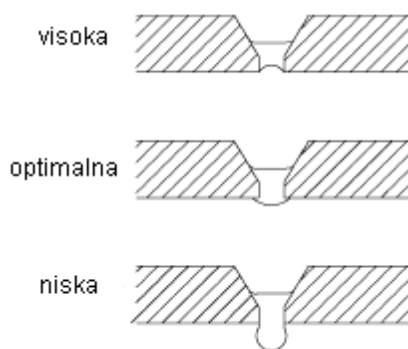
Slika 3.3 Utjecaj pozadinske struje na geometriju zavara [8]
