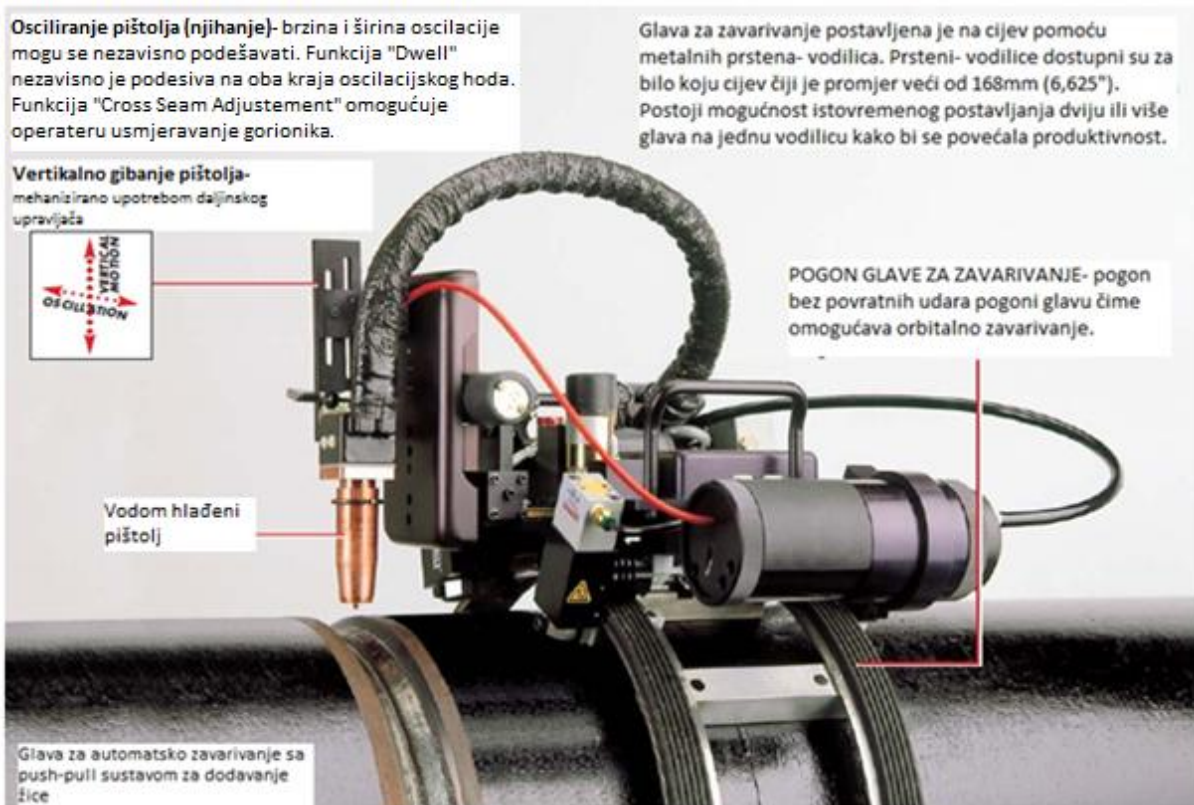
Slika 6.2 Automatska glava za zavarivanje model 609 [12]
