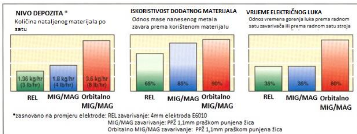
Slika 6.1 Dijagram količine rastaljenog materijala [12]
