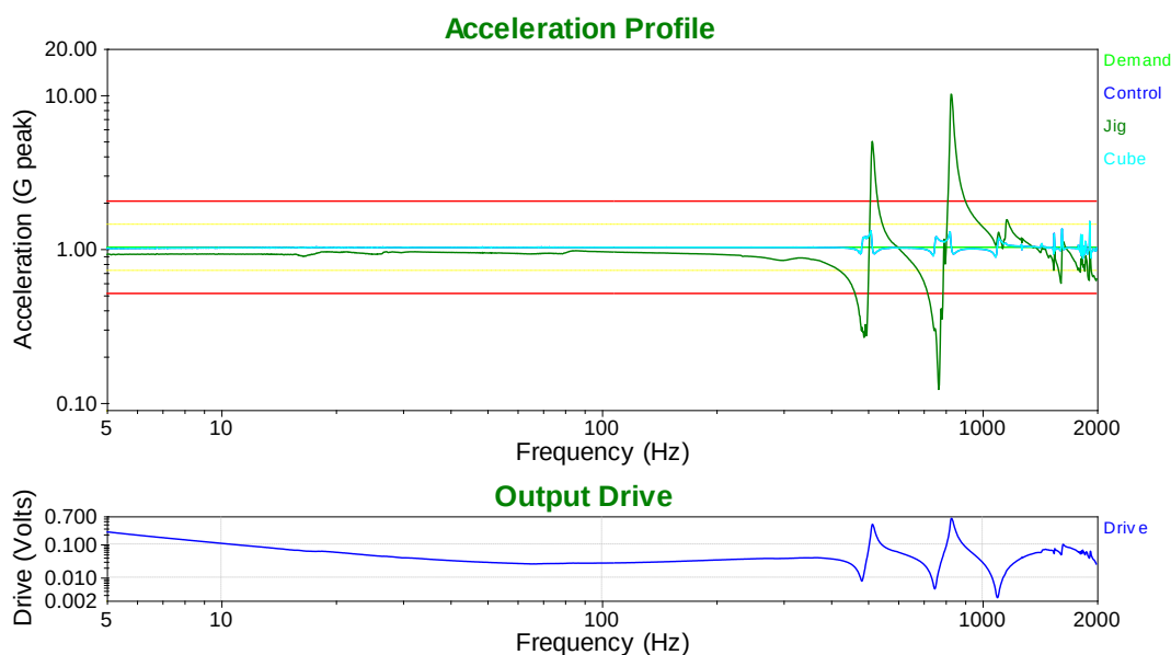
Slika 24. Frekvencijski profil
