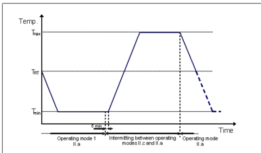
Slika 20. Temperaturni profil
