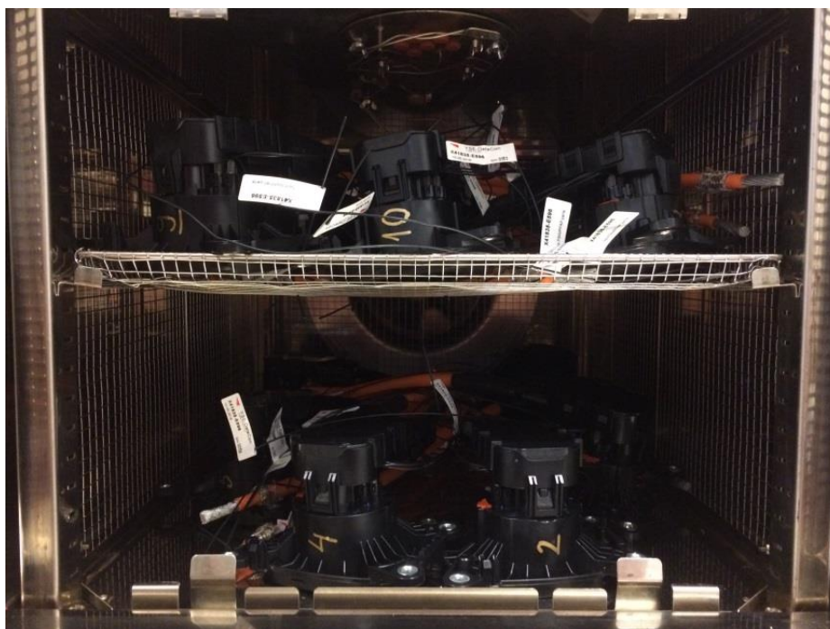
Slika 16. Ispitni predmeti položeni unutar šok komore
