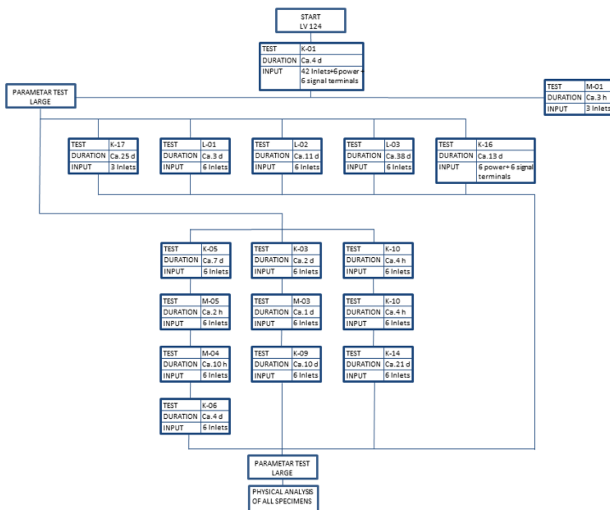
Slika 9. Dijagram aktivnosti provođenja ispitivanja (Flow chart)
