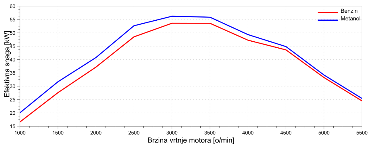
Slika 4.14. Krivulje snage pri punom opterećenju
