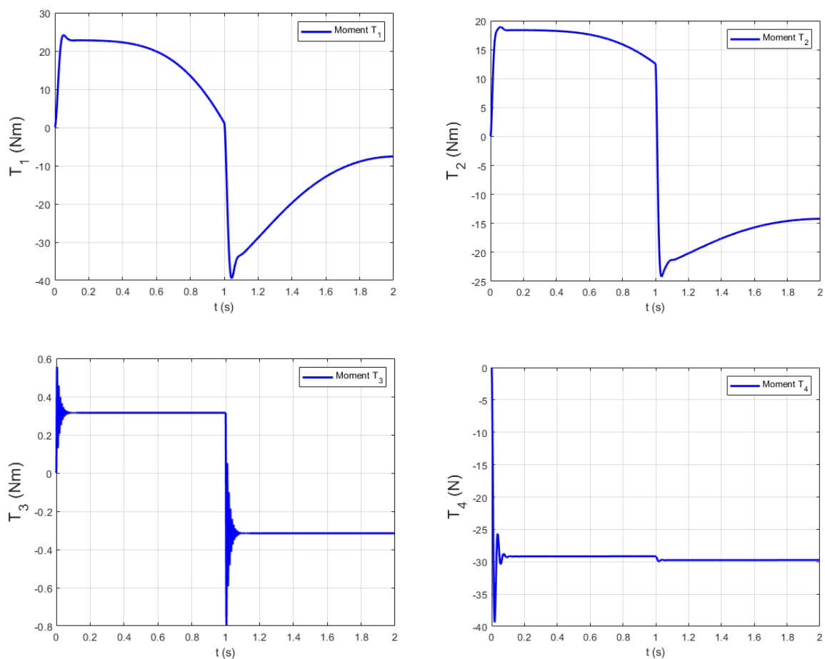
Slika 41. Odzivi momenata robota s upravljanim koordinatama PD regulatorom na paraboličnu pobudu
