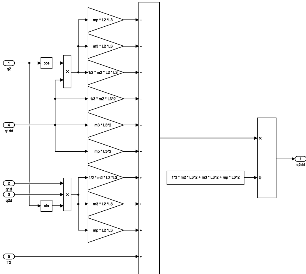
Slika 8. 2. upravljana koordinata
