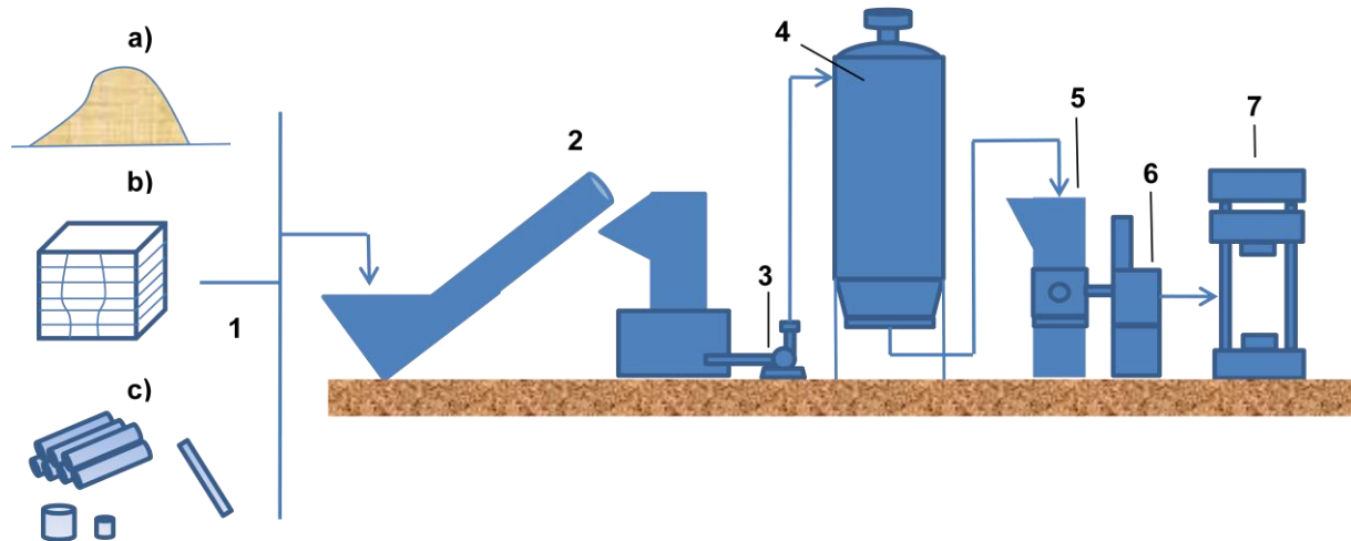
Slika 4.4. Postrojenje za pravljenje izravno prešanih otpresaka od otpadne plastike a - granulirani smećak, b - kompoziti, filmovi, folije, runo, c - kruta plastika, 1 - plastični otpad, 2 - usitnjavalica, 3 - mehanička ili pneumatska dobava, 4 - silos, 5 - plastifikator s istiskivalicom, 6 - volumno doziranje (obujmena odmjera) plastifikata, 7 - automatska dobava preša za izravno prešanje [1]
