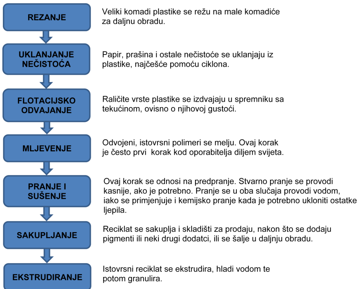
Slika 4.2. Shema mehaničkog recikliranja plastičnog otpada [13]
