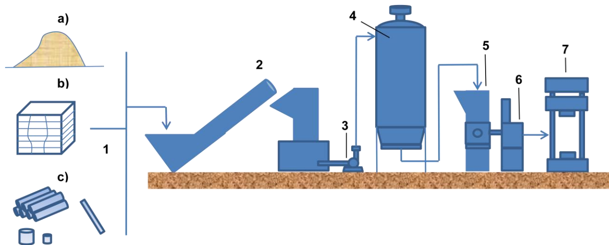
Slika 4.4. Postrojenje za pravljenje izravno prešanih otpresaka od otpadne plastike a - granulirani smećak, b - kompozitni materijali, filmovi, folije, runo, c - kruta plastika, 1 - plastični otpad, 2 - usitnjavalica, 3 - mehanička ili pneumatska dobava, 4 - silos, 5 - plastifikator s istiskivalicom, 6 - volumno doziranje (obujmena odmjera) plastifikata, 7 - automatska dobava preša za izravno prešanje [1]
