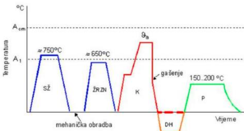
Slika 2. Cjelokupni postupak toplinske obrade čelika EN DIN 100Cr6[4]
