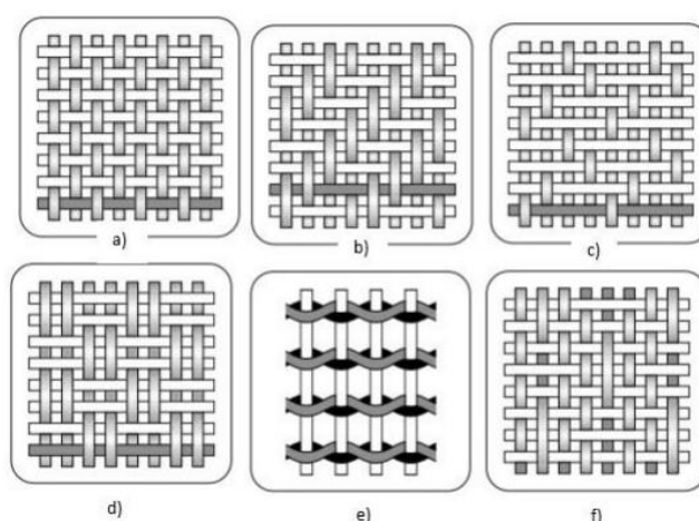
Slika 7. Tipovi tkanja : a) platno (obično), b) atlas, c) keper, d) tkanje košarice, e) leno, f) inačica običnog tkanja
