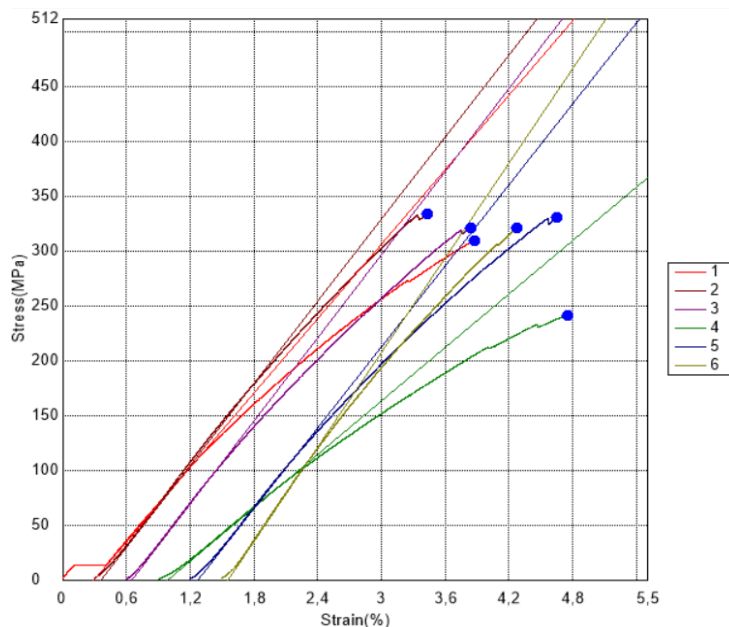
Slika 19. Dijagram naprežanje – istežanje dobiven savojnim ispitivanjem za kompozit epoksid / staklo i lan
