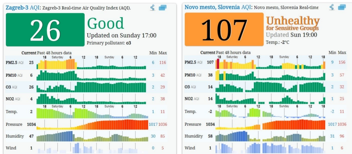
Slika 4. Usporedba indeksa kvalitete zraka s prikazom koncentracije onečišćujućih tvari u Zagrebu (lijevo) i Novom Mestu (desno) u poslijepodnevnom satima 5. veljače 2023. [11]
