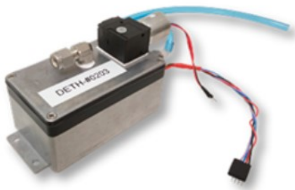
Slika 12. "Mini sniffer" sensor tvrtke Explicit [26]
