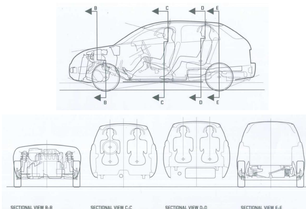
Slika 13. Presjeci glavnih dijelova vozila [2]
