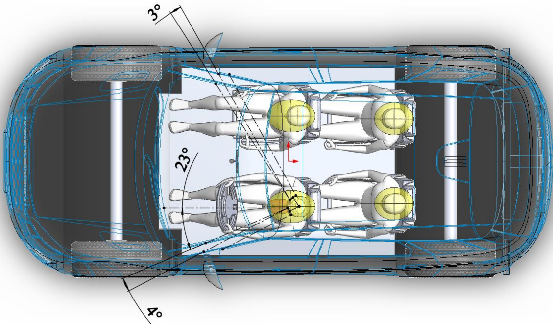
Slika 42. Kutovi zaklanjanja pogleda vozača
