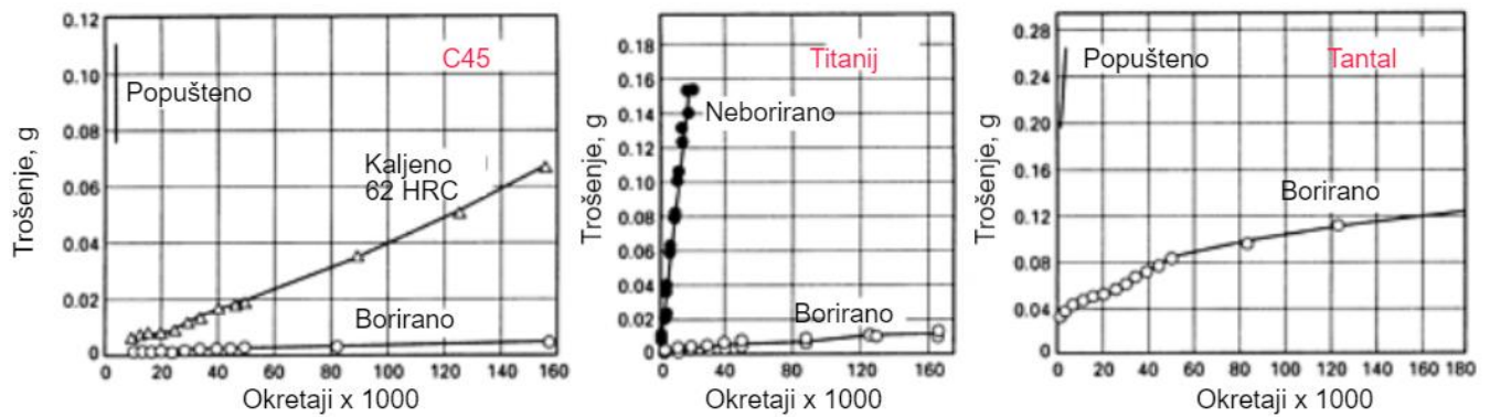
Slika 2. Utjecaj boriranja na trošenje čelika C45, titanija i tantala [4]
