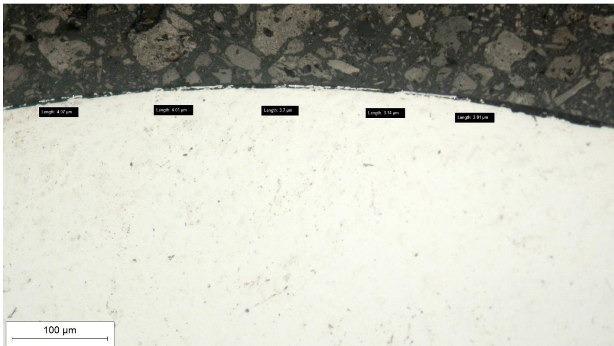
Slika 36. Uzorak 4, boriran na T = 900\text{ °C}/1\text{h} , povećanje 200x, nagriženo u 3 %-tnom NITAL-u
