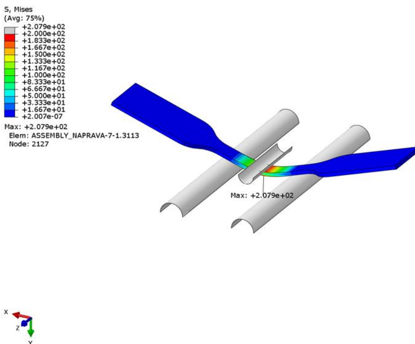
Slika 48. Raspodjela napreznja na epruveti debljine 0,5 mm – materijal dobiven eksperimentalnim ispitivanjima
