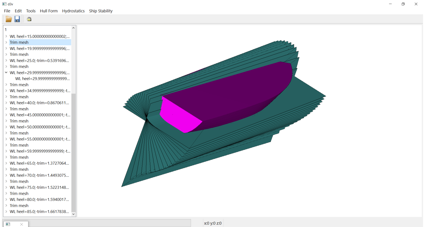
Slika 18. Prikaz ravnina vodne linije pri određenim nagibima broda
