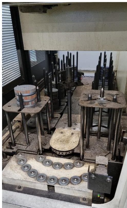
Slika 24. Robotska doprema sirovaca
