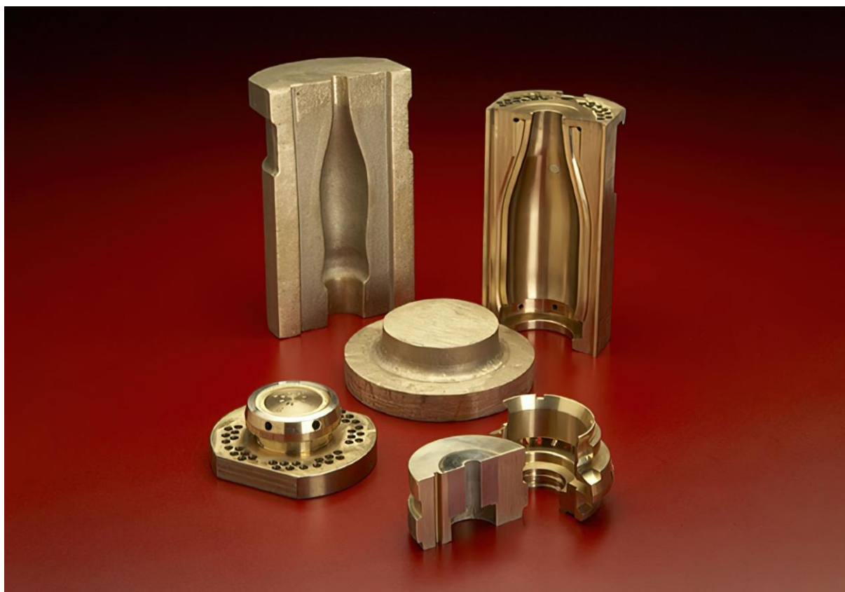
Slika 6. Staklarski alati
