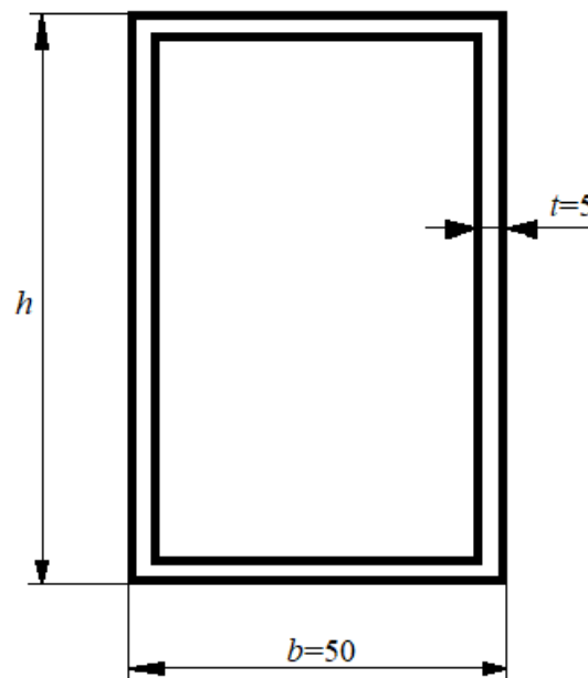
Slika 21 Dimenzije poprečnog presjeka pravokutne cijevi
