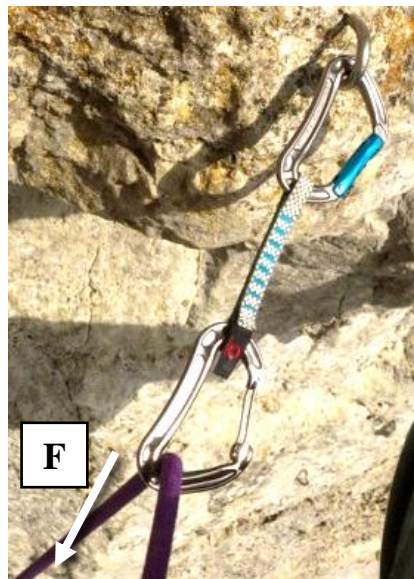
Slika 17. Opterećeni komplet [24]
