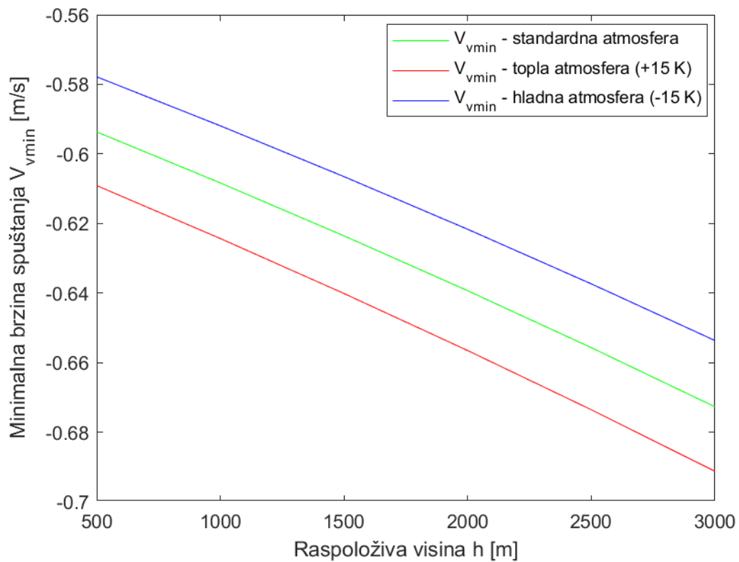
Slika 24. Minimalna brzina spuštavanja za režim najveće istrajnosti u ovisnosti o raspoloživoj visini leta i usporedba za različita stanja atmosfere
