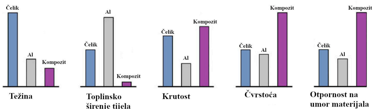
Slika 1. Usporedba svojstava kompozita s konstrukcijskim čelikom i aluminijem [2]
