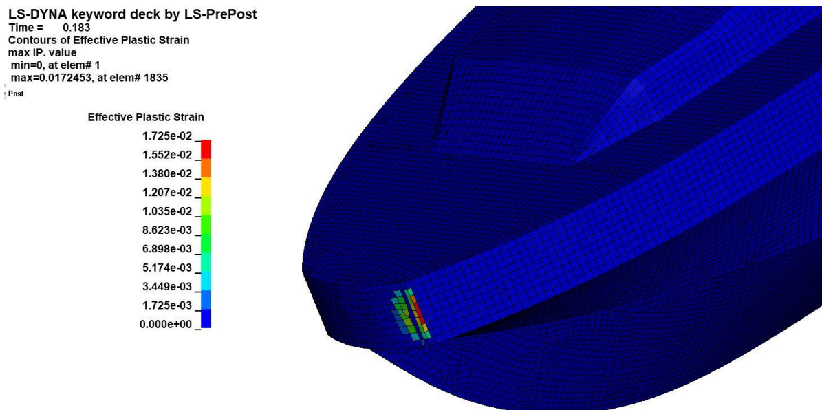
Slika 49 Prikaz plastičnih deformacija pri frontalnom sudaru pod kutem od 30°, brod sa PE bokoštanicima, brzina 5,5 čv
