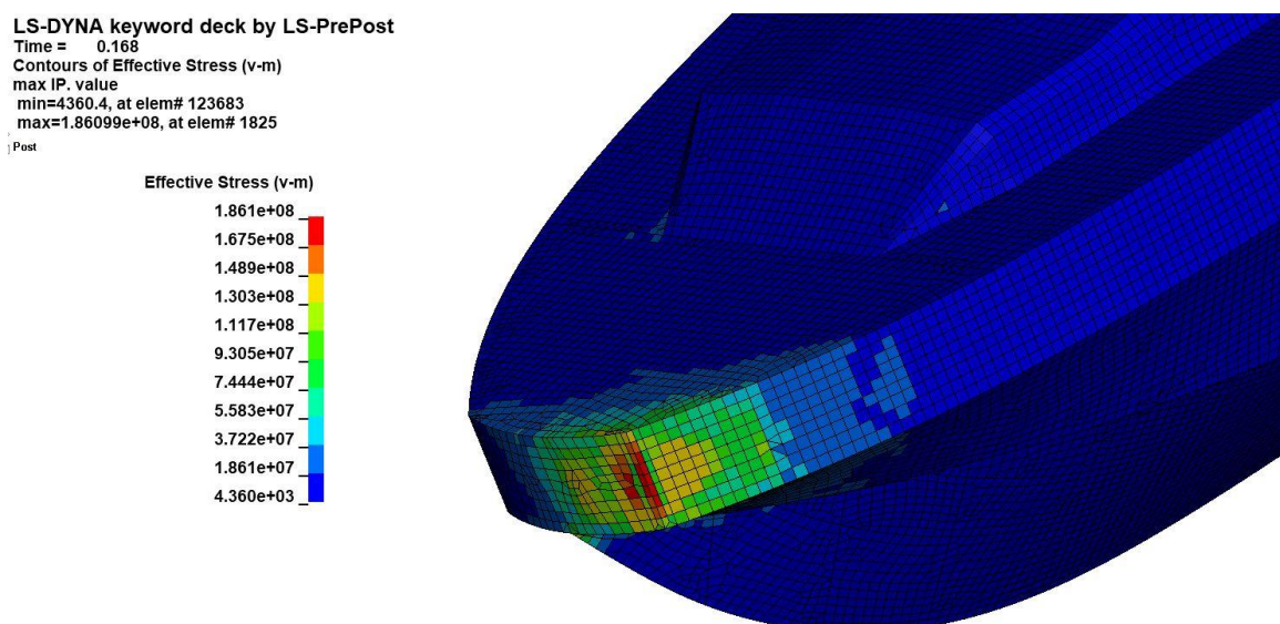
Slika 50 Prikaz Von Mises naprezanja pri frontalnom sudaru pod kutem 30°, brod sa PE bokoštanicima, brzina 5,5 čv
