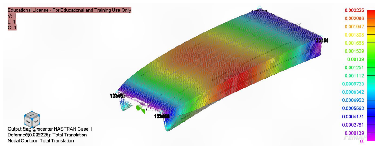
Slika 88. Prikaz deformacija
