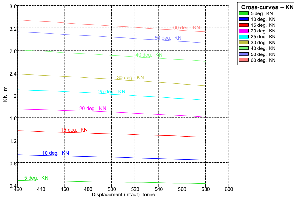
Slika 14 KN krivulje
