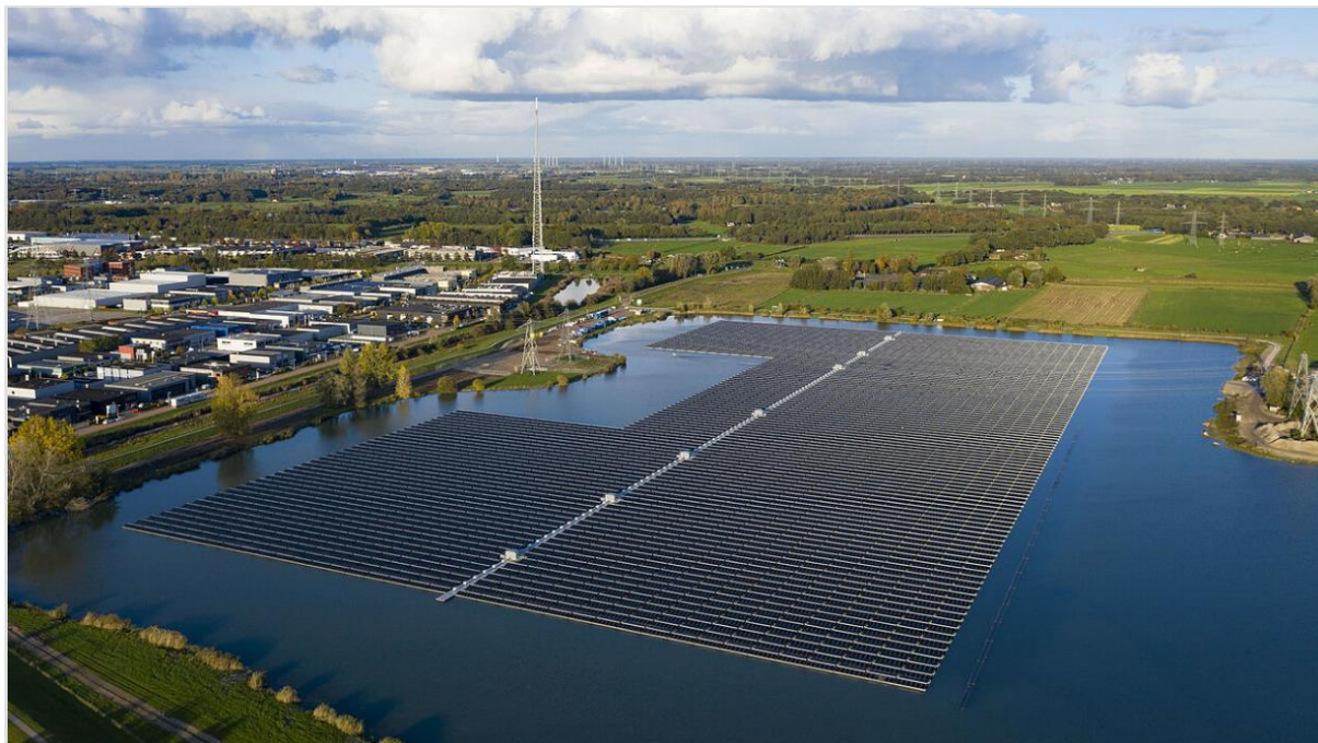
Slika 3.7 Sekdoorn FPV sustav u Nizozemskoj snage 14,5 MW [19]
