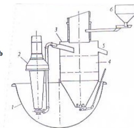
Slika 5. Harrisov uređaj [6]
