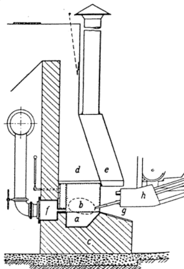
Slika 3. Newnamova peć [6]
