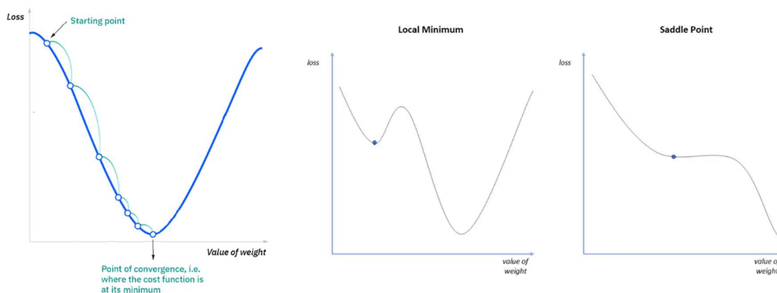
Slika 5. Funkcije pogreške
