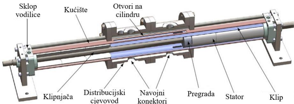
Slika 33. Ekspander s kotrljajućim klipom [124]
