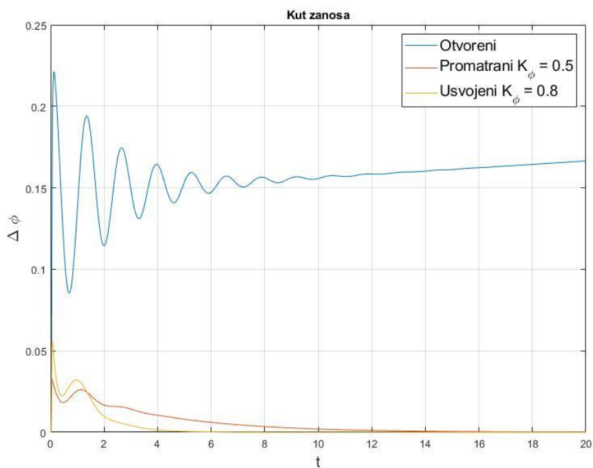
Slika 7.7. Odziv kuta zanosa \phi
