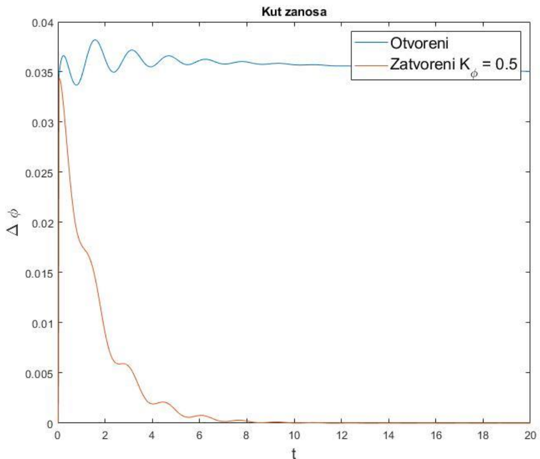
Slika 7.4. Povratna veza po kutu zanosu \phi
