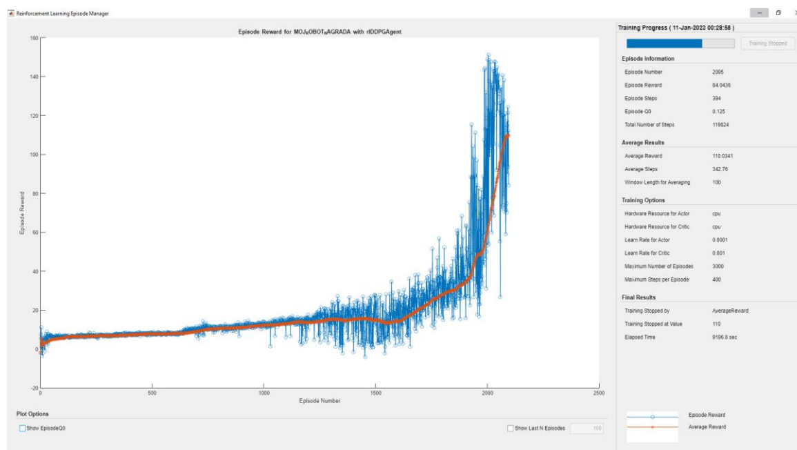
Slika 66 graf s nagradama tokom treniranja Agenta s izmjenama u nagradnoj funkciji
