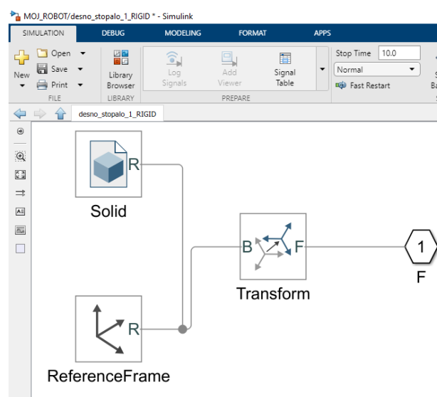
Slika 19 Podsustav “desno_stopalo_1_rigid“
