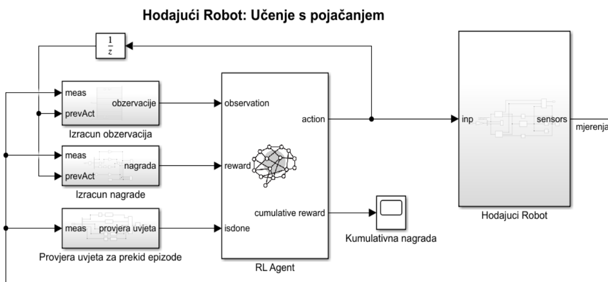
Slika 53 Model za implementaciju učenja s pojačanjem
