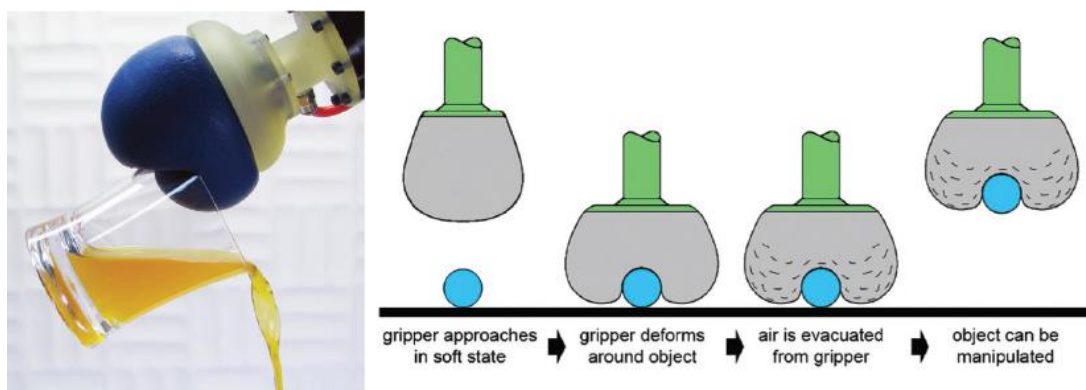
Slika 7. Granularno nabijanje, [5]
