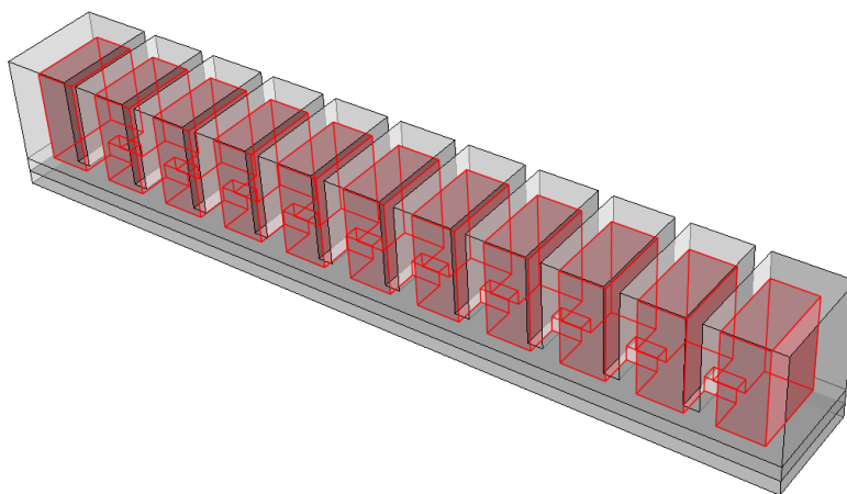
Slika 29. Komore aktuatora na koje djeluje unutarnji tlak
