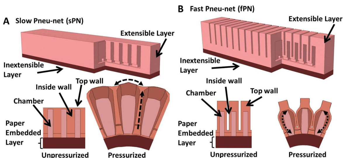
Slika 6. Fluidički elastomerni aktuatori (FEA), oblik A i B, [12]
