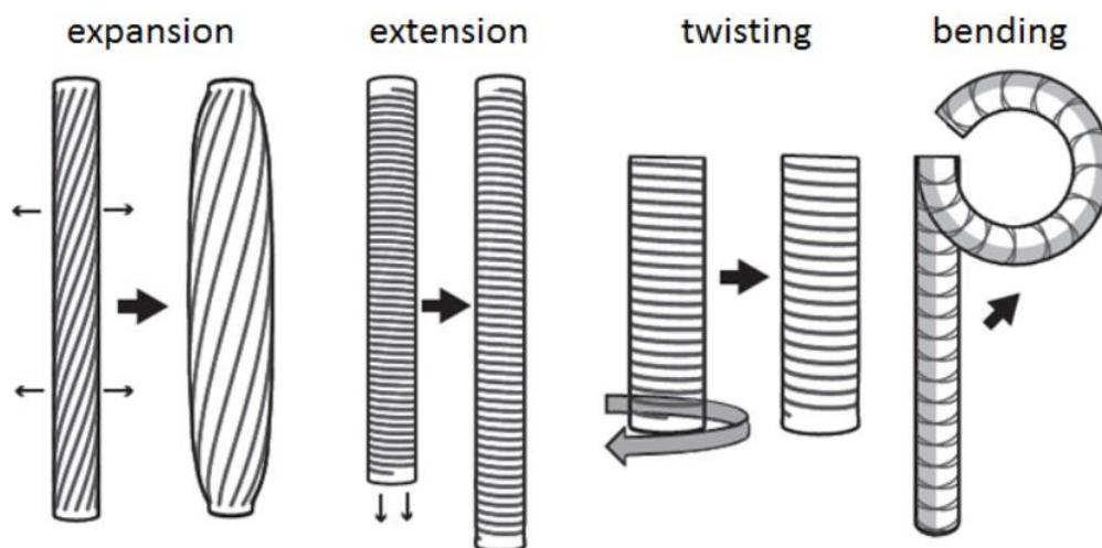
Slika 13. Utjecaj smjera namatanja niti na gibanje aktuatora, [13]
