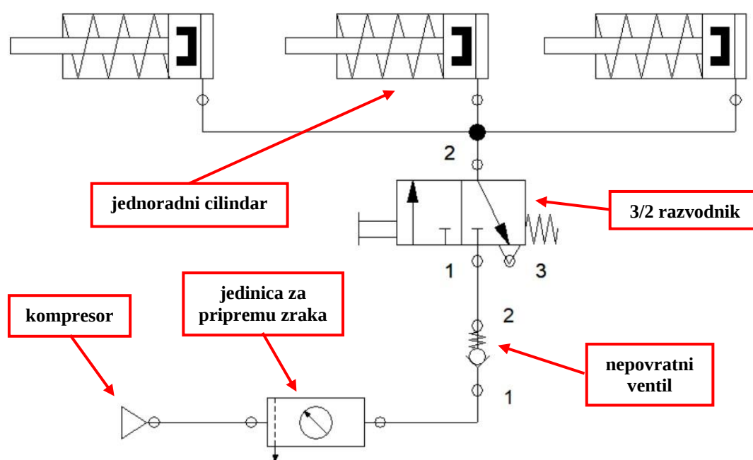
Slika 27. Pneumatska shema
