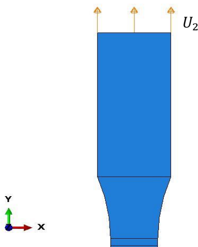
Slika 27. Opterećenje epruvete zadavanjem pomaka
