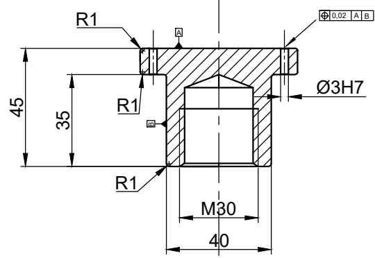
Presjek B-B
