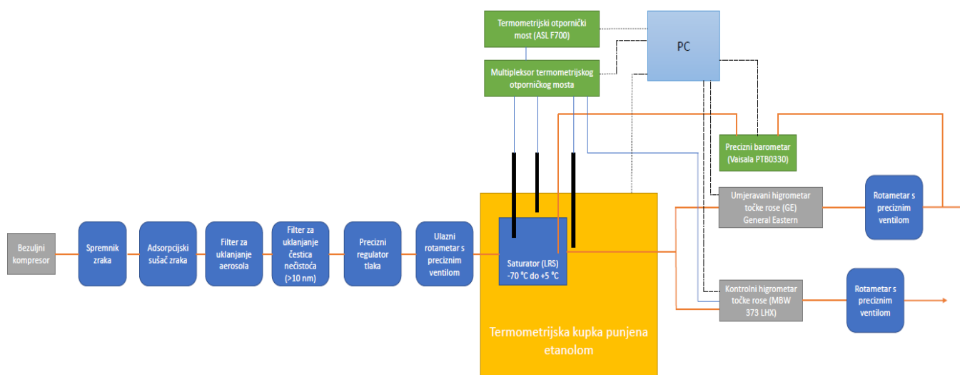
Slika 9. Shema mjerne linije za temperaturno područje od -25 °C do 1 °C
