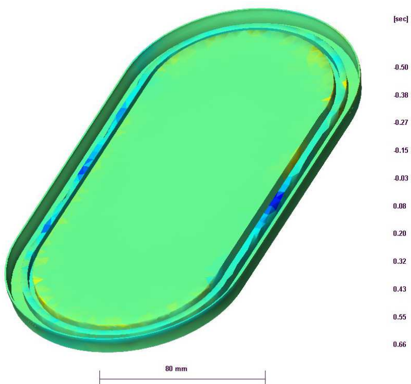
Slika 6.6: Razdioba vremena hlađenja
