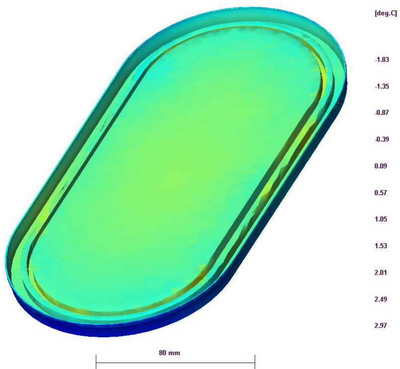
Slika 6.5: Razdioba površinskih temperatura
