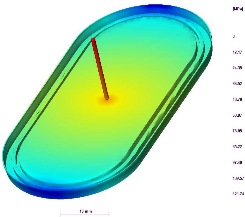
Slika 6.2: Tlak ubrizgavanja
