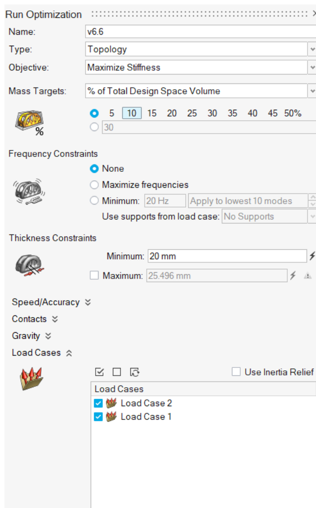
Slika 43: Maksimiranje krutosti
