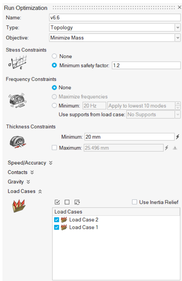
Slika 44: Minimiranje mase
