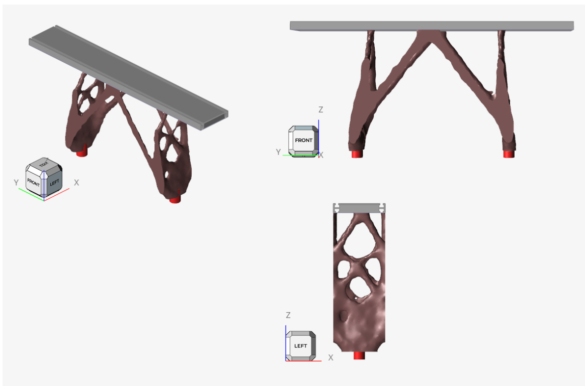
Slika 45: Maksimiranje krutosti (5%)
