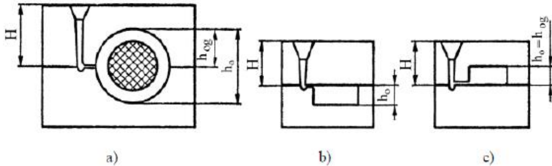
Slika 29. Visina taline ovisi o smještaju modela u kalup i lijevanju: a) sa strane, b) odozgo, c) odozdo
