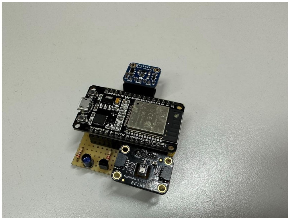
Slika 39. Izrađeni uređaj
