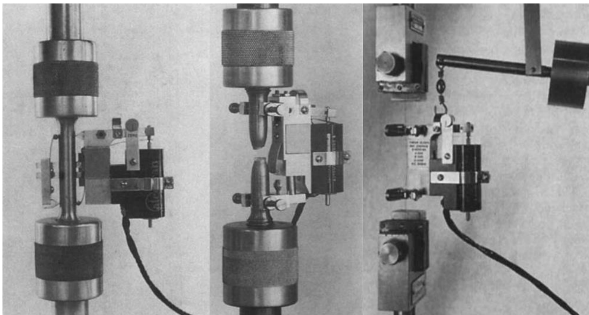
Slika 10. LVDT ekstenzometar prilikom ispitivanja na različitim uzorcima i u trenutku loma [4]
