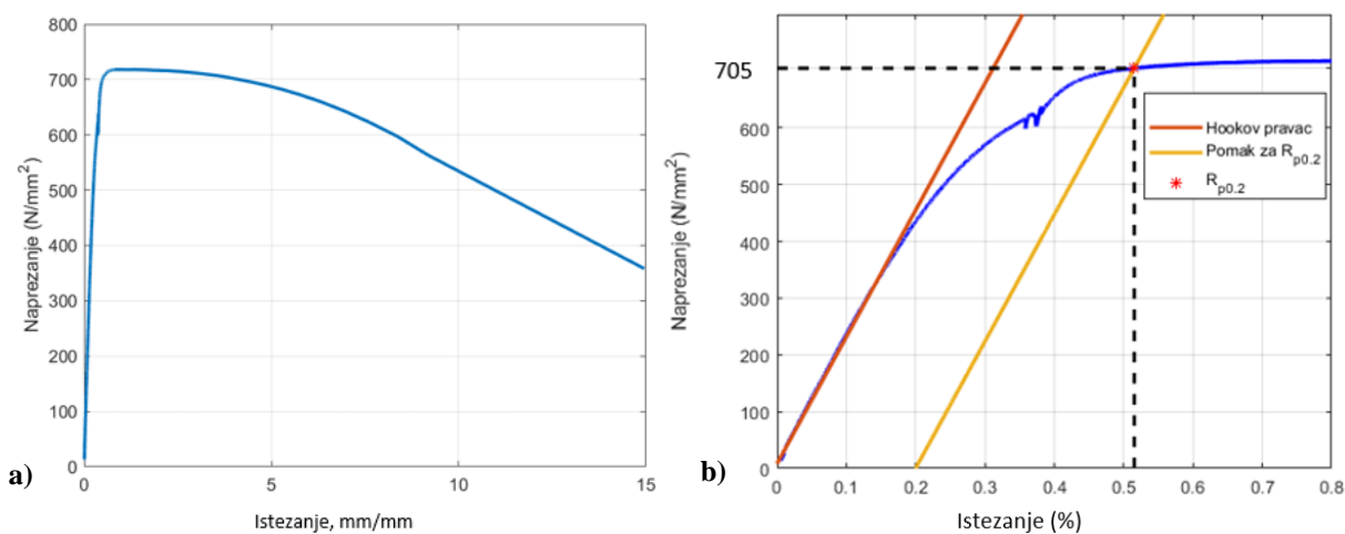
Slika 38. \sigma - \varepsilon dijagram (a) s istaknutim područjem elastičnosti (b) za frekvenciju ispitivanja 20 Hz, čelik 50CrV4
