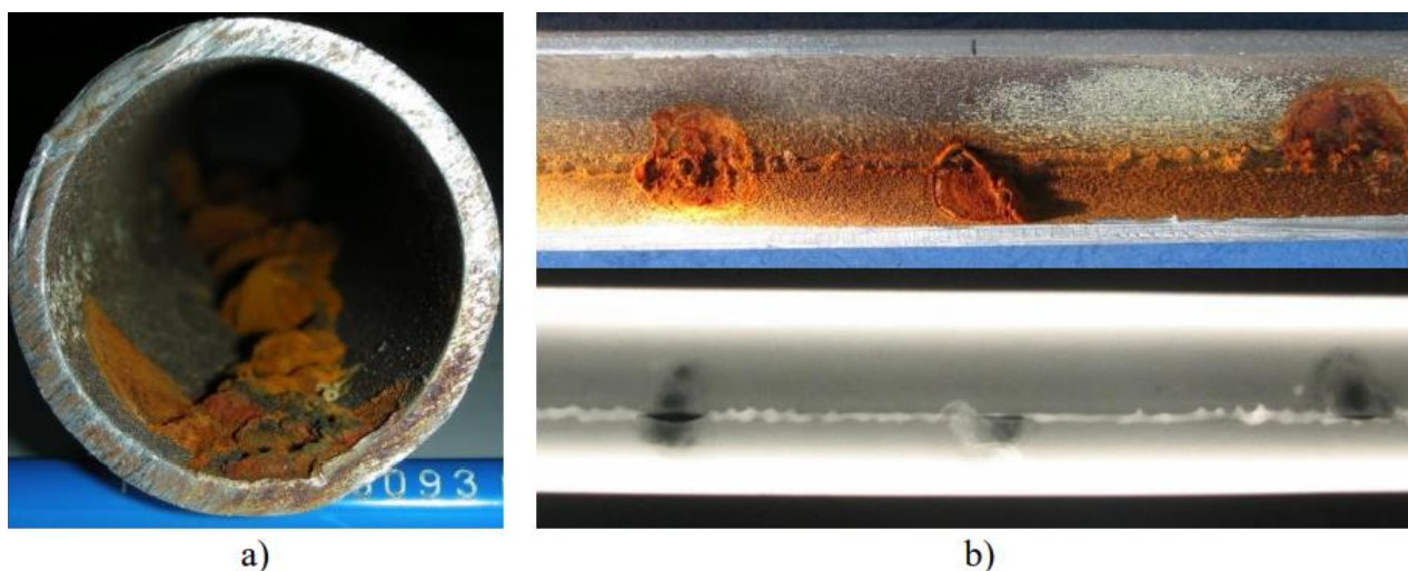
Slika 11. Rovna korozija uzduž zavora ispod nakupina hrđe [10]
