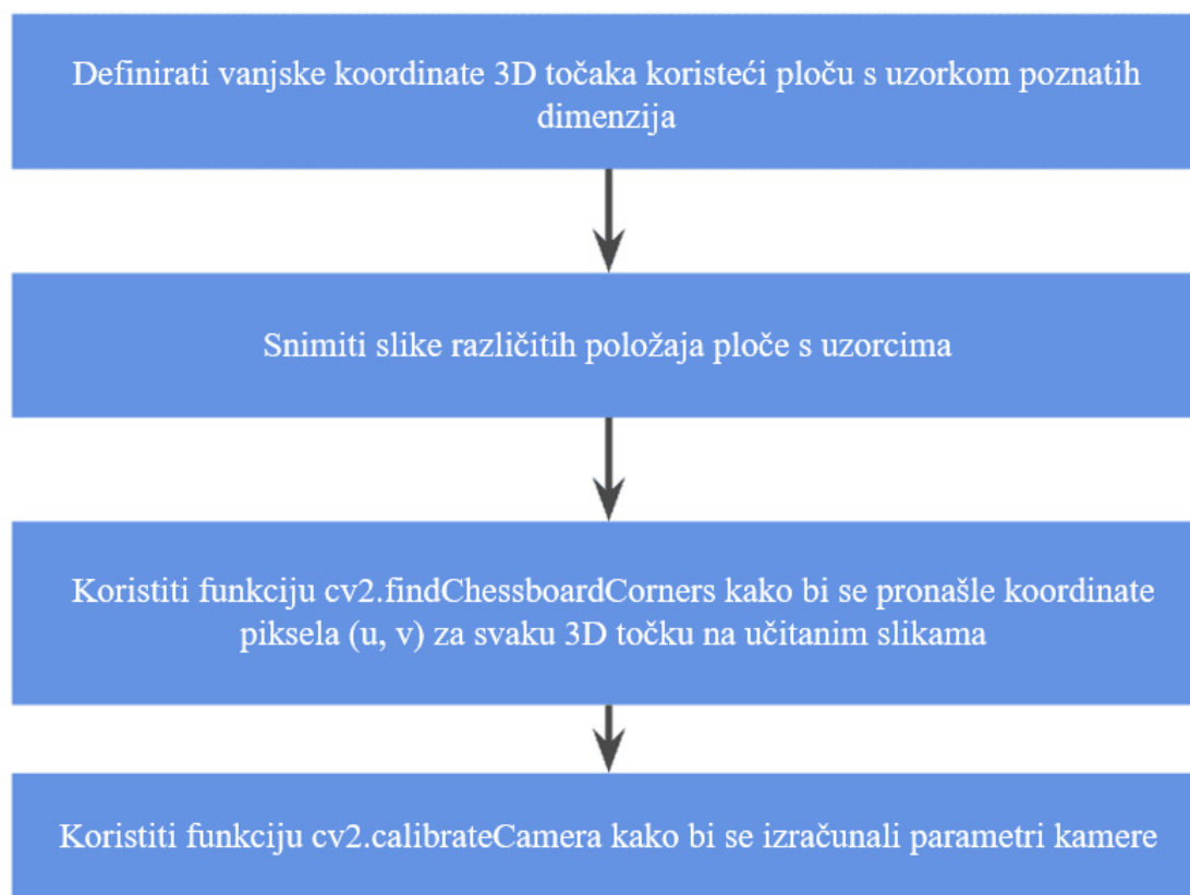
Slika 4.21. Dijagram toka kalibracije kamere
