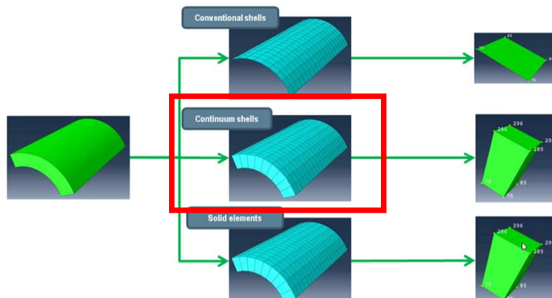
Slika 43. 3D ljuskasti konačni elementi [47]
