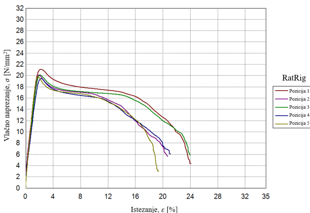
Slika 4.20 Graf \sigma - \epsilon za ispitna tijela ispisana RatRig V-Minion običnom mlaznicom
